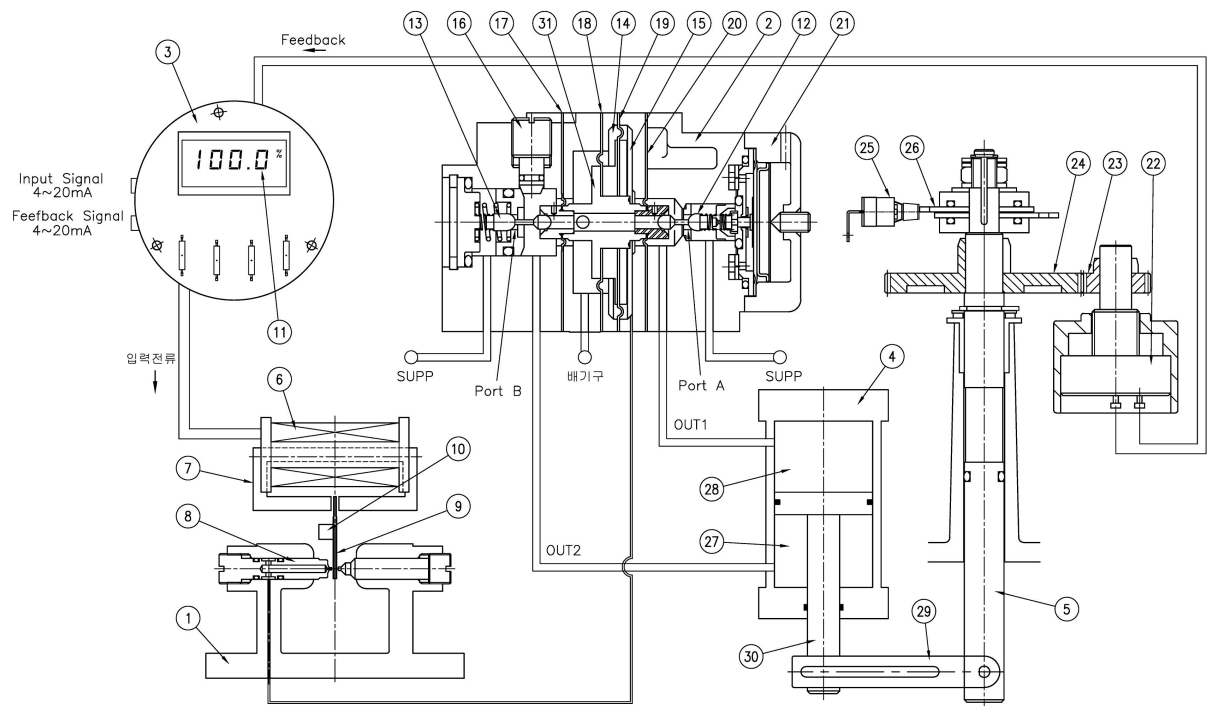
그림 2-3 : 동작원리도
