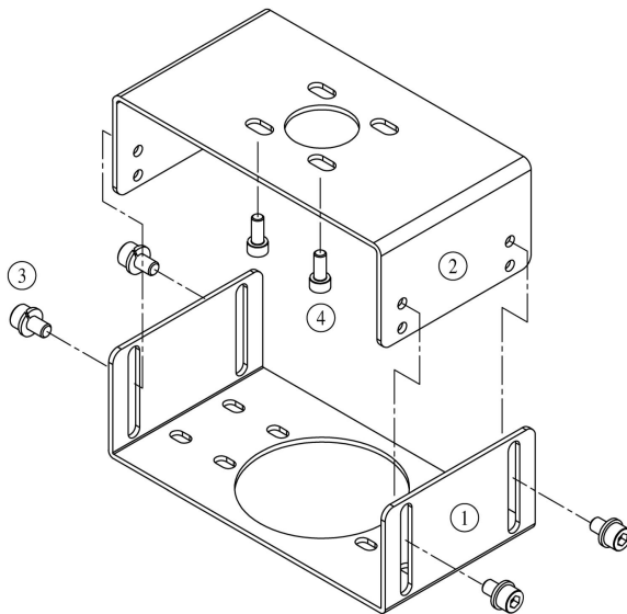
그림 3-9 : 로타리 포지셔너 설치용 브라켓 세트
