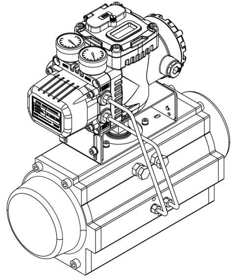
그림 4-4 : 복동식 로터리 액츄에이터
