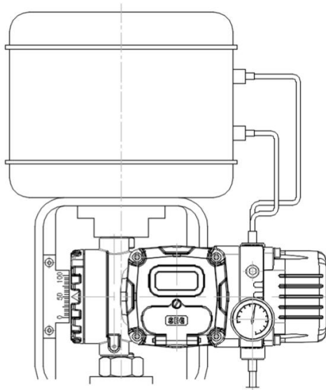
그림 4-3 : 복동식 리니어 액츄에이터
