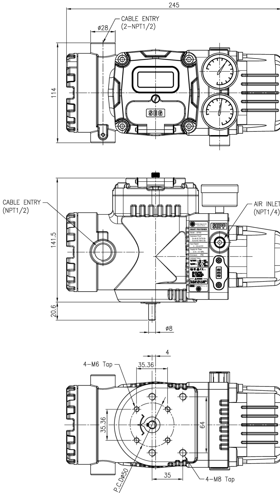
그림 2-5 : SP760 기본형
