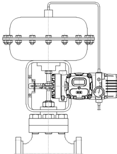
그림 3-1 : SP760 설치예
