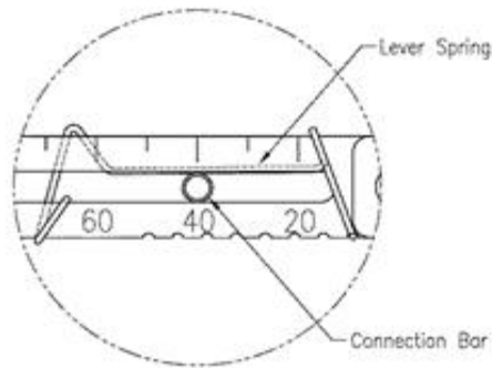
그림 3-4 : 레버와 스프링 사이에 연결봉 삽입방법
